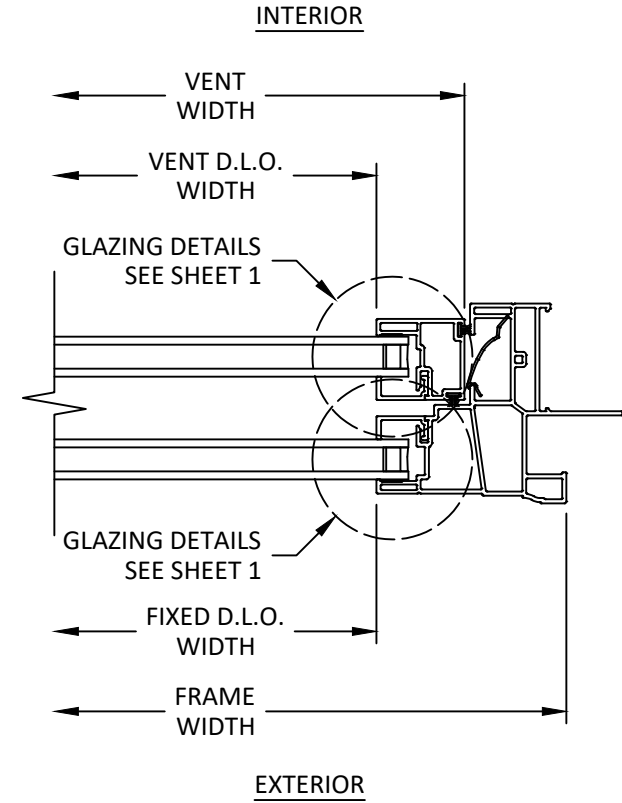
E 4 HORIZONTAL SECTION JAMB
