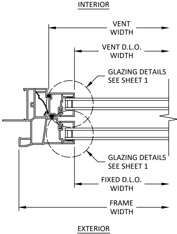
D 4 HORIZONTAL SECTION JAMB
